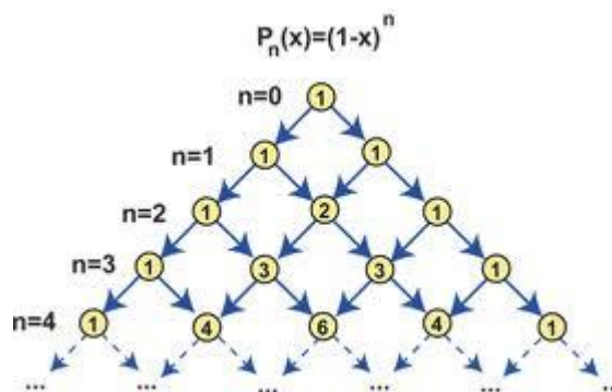
Рисунок 3 – Перші 5 рядків трикутника Паскаля ( n = 0, 1, \dots, 4 ) [16]
