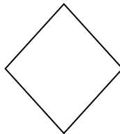
Рисунок 2 – Приклад лінгвістичного фрактала [16]
